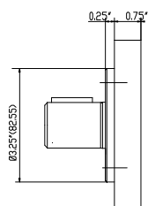
BM5 Motor Flange
